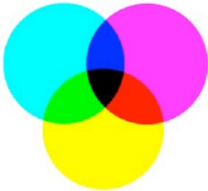
CMYK
